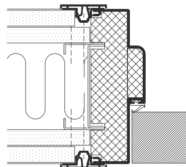
Tür in DEKO PF Systemwand Aluminiumverkleidung Typ ASPD
