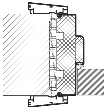
Tür in Betonwand Aluminiumverkleidung Typ ASIF
