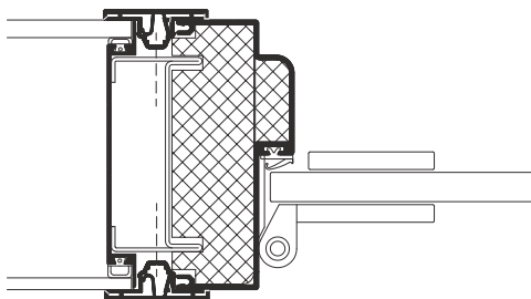
Ganzglastür in DEKO GV Glaswand Aluminiumverkleidung Typ ASPD
