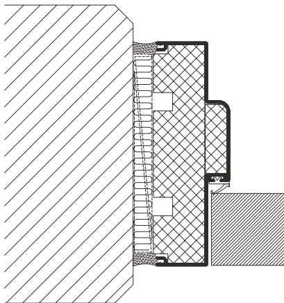
Tür in Betonwand - Fugenverbindung
