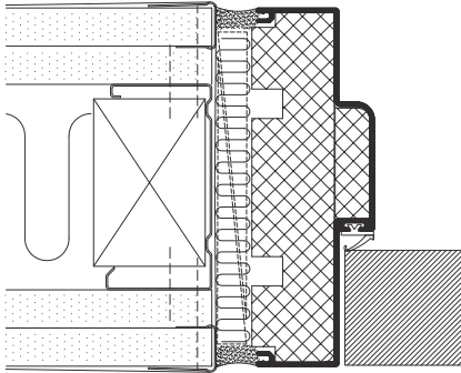
Tür in Gipskartonwand - Fugenverbindung
