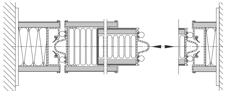
Wandanschluss
