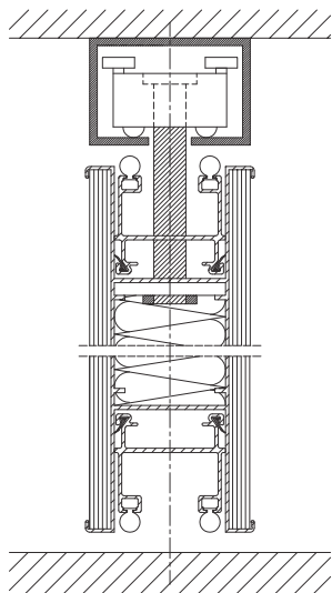
Decken-/Bodenanschluss
