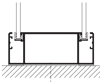
Bodenverbindung
