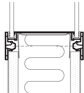
Vertikalschnitt Gipsplatten-/Glasverbindung
