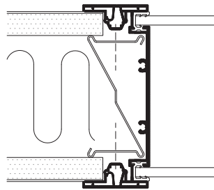
Horizontalschnitt Gipsplatten-/Glasverbindung
