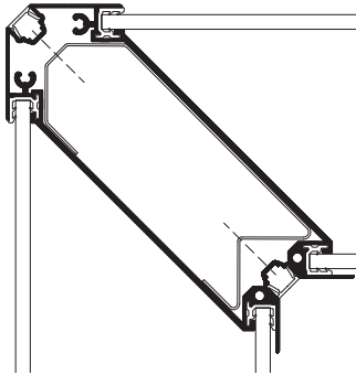
90° Ecke
