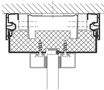
Deckenanschluss
